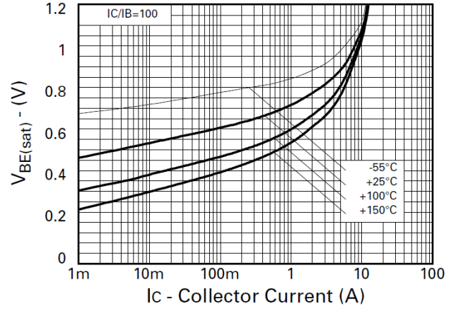
Fig.8 V_{BE(sat)} \text{ v } I_C
